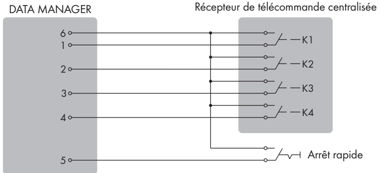
Figure 7 : Raccordement d'un récepteur de télécommande centralisée
